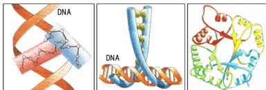
ヘリックス・ターン・ヘリックス ロイシンジッパー \alpha/\beta -バレル
