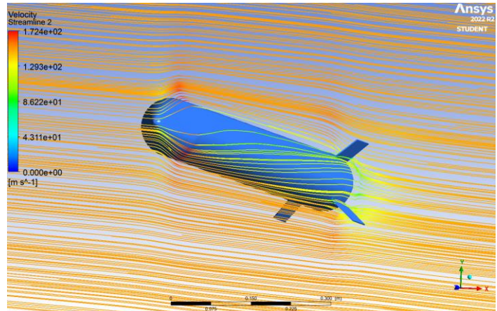
数値流体解析(CFD解析)
